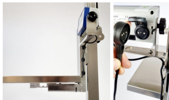
Plattformsvåg kontrollvåg. Laddas med 12 volt magnetkontakt. Spolbar. IPX5.
